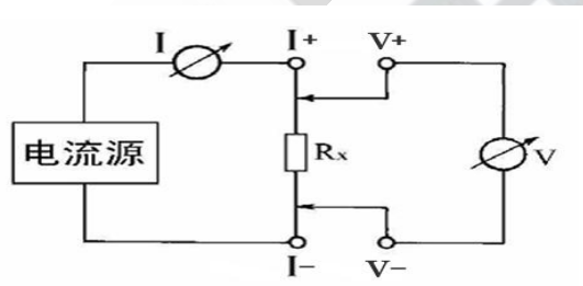
图二 测试原理图
