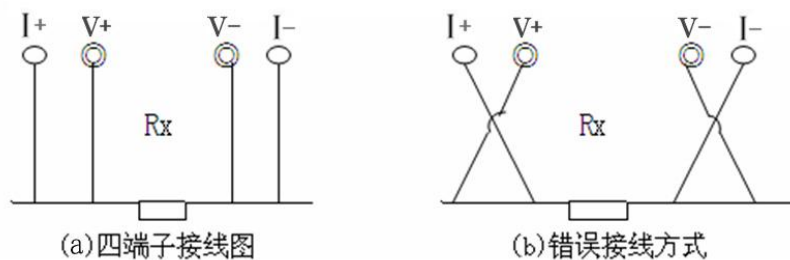
图三 四端子接线图
