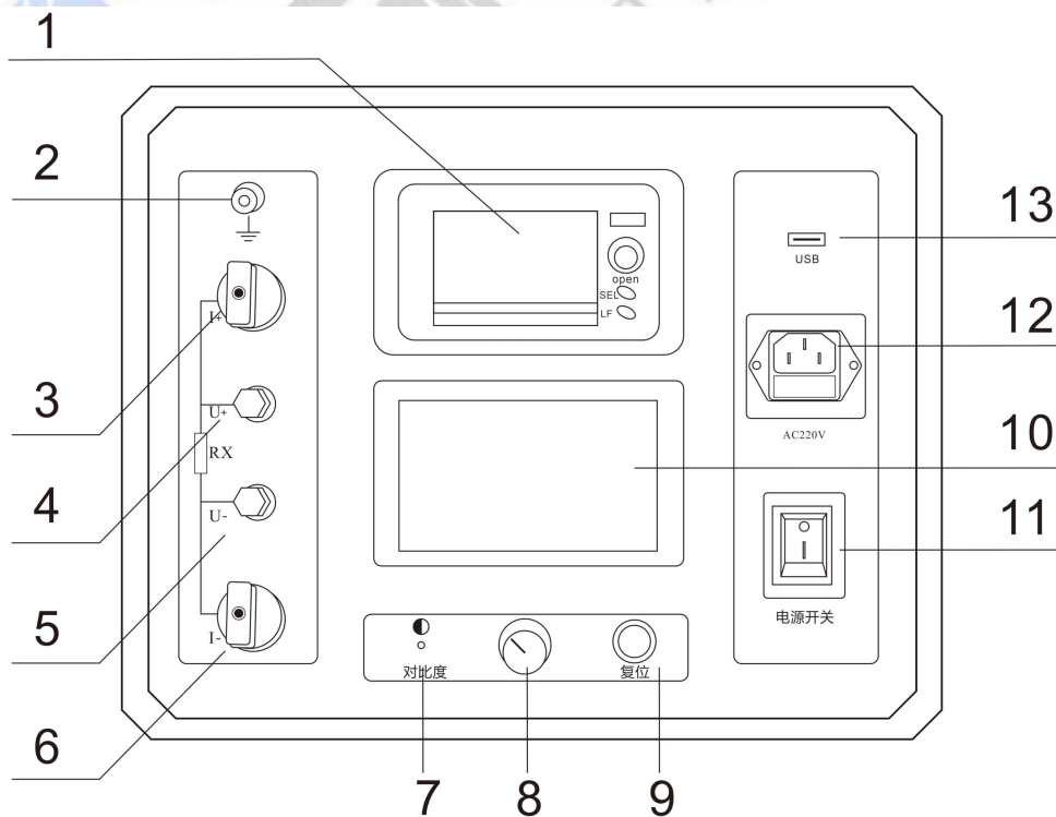
图一面板结构图
